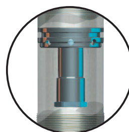
Überdruckventil / Blow off valve: LL-23 / LL-24 / LL-25
