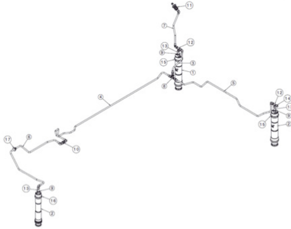
Beispiel-Planung für 3 Airjacks
