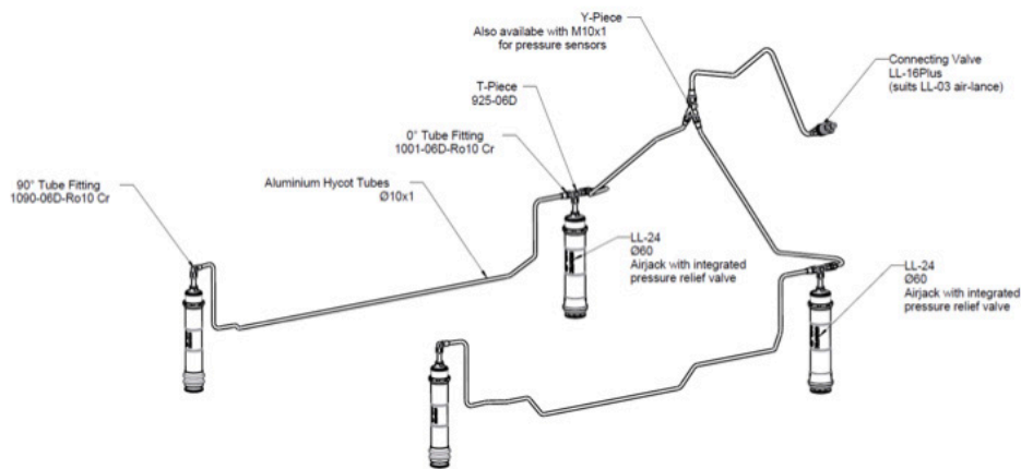
Beispiel-Planung für 4 Airjacks
